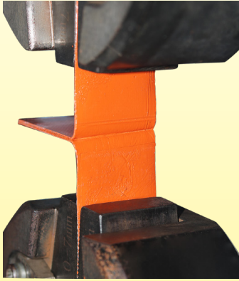
Vulkanisierte Probe vor der Ablösungsprüfung
